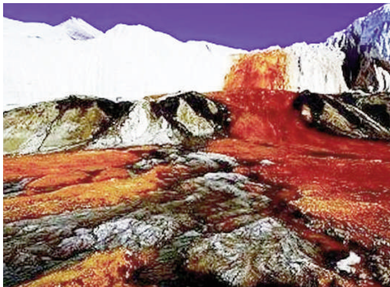
Salmuera rica en hierro se oxida al salir del glaciar.
