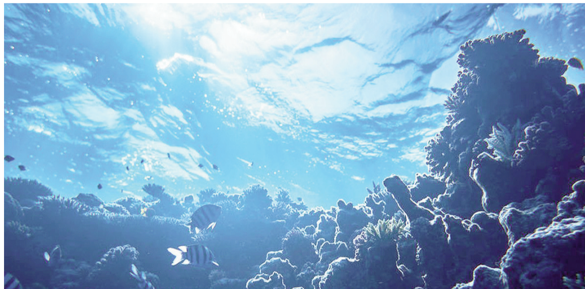
La nieve marina transporta carbono desde la superficie del océano hasta las profundidades, donde puede quedar retenido durante siglos y ayuda a regular el clima.
